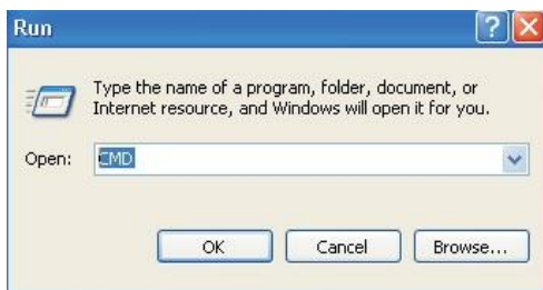
Рис. 3-4 Командное окно
